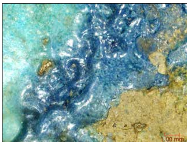
Figura 4. Dettaglio delle fratture/discontinuità nella zona di contatto, microscopio digitale USB 20x
